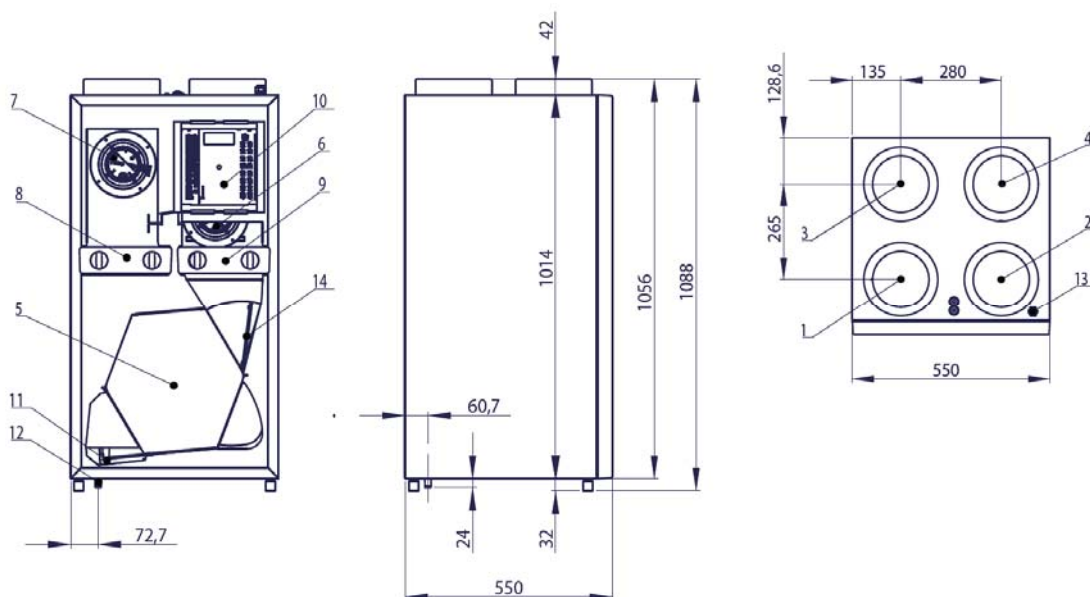
12. Condensaat afvoer
